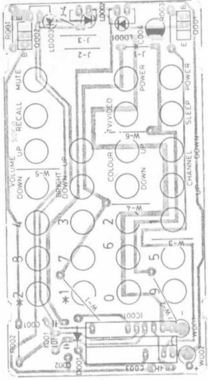
底视图
