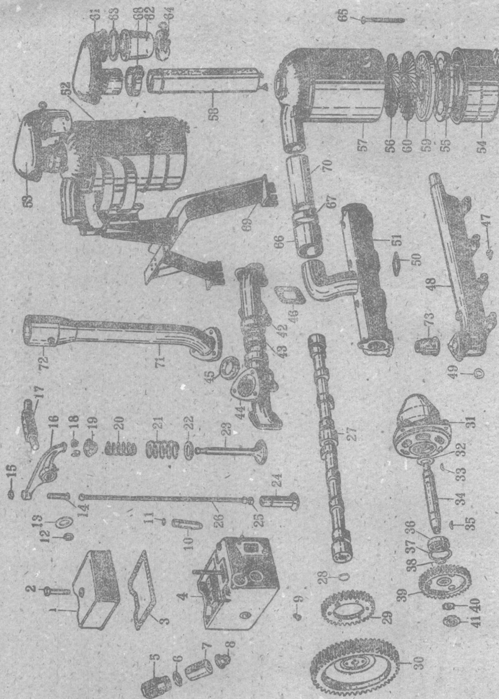
图 1 气缸盖、凸轮轴、吸气管、排气歧管、油浴式空气滤清器、燃油泵驱动部分
