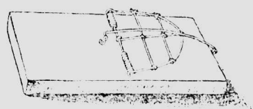
图 4 用木板、彈簧或竹子制成鼠夾，裝上食物，支在鼠洞附近的牆边上，可以捕打兩面来的老鼠。
