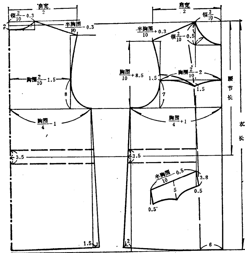
女小学生上衣裁剪图
