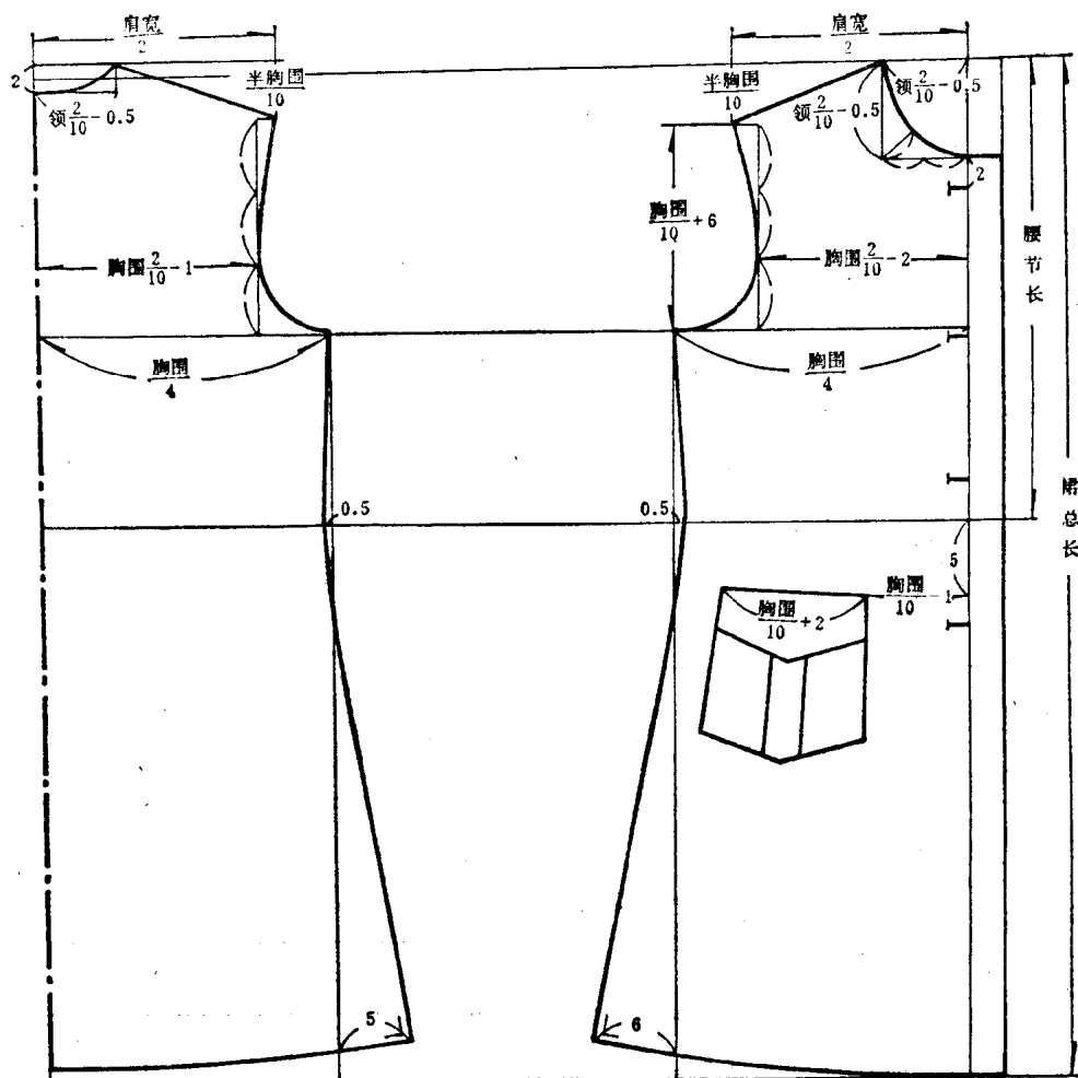
女小学生连衣裙裁剪图
