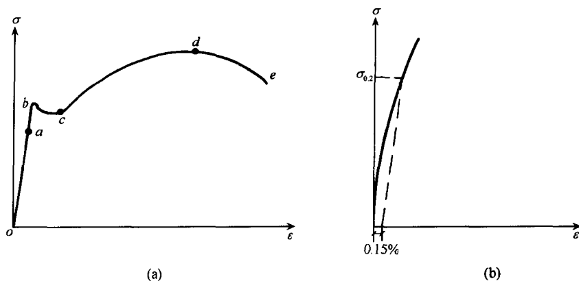
图 2.2 钢筋的应力-应变关系
