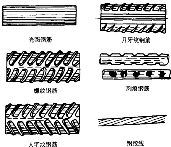
图 2.1 各种钢筋的形式
