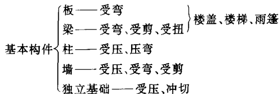
图 1.1 基本构件
