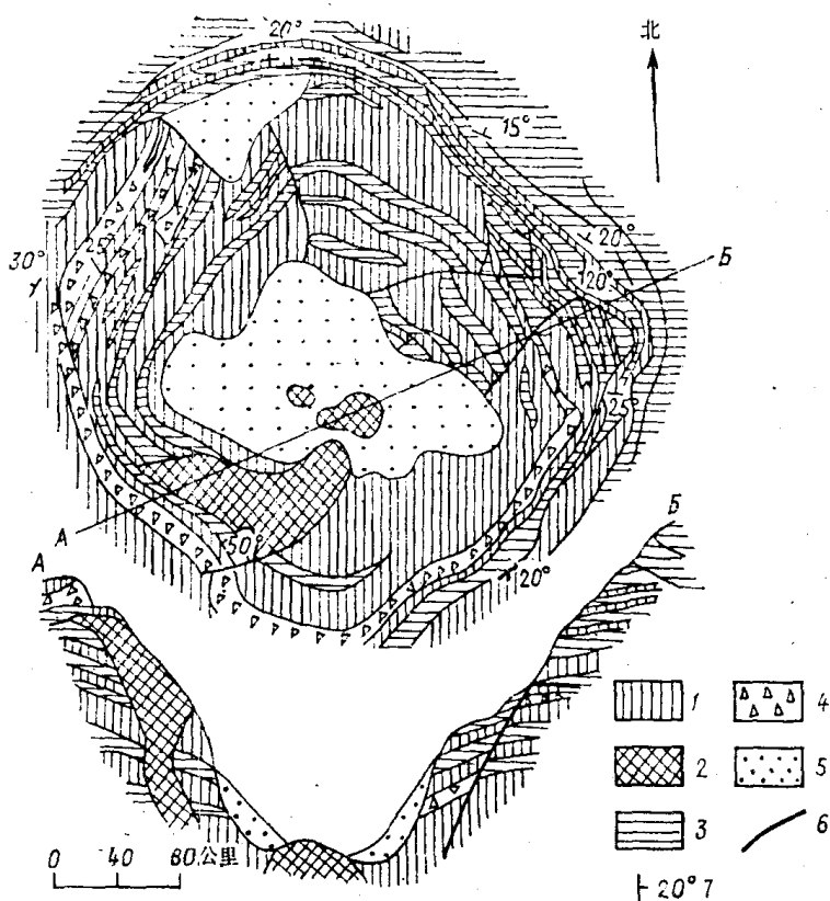
图 4 阿瓦恰火山口的结构略图
