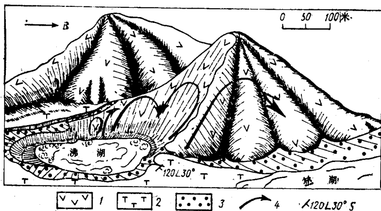
图3 戈洛夫宁纳火山的现代火山口地区
