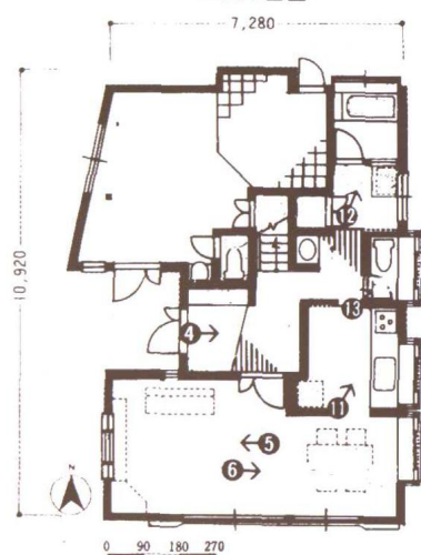
一层平面图
