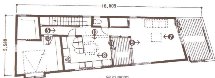
一层平面图
