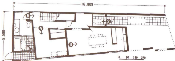
二层平面图
