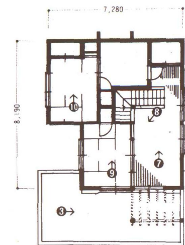
二层平面图
