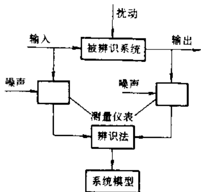
图 1-1 系统辨识问题方框图
