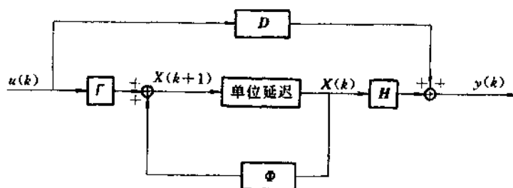
图 1-6 系统的状态空间表达
