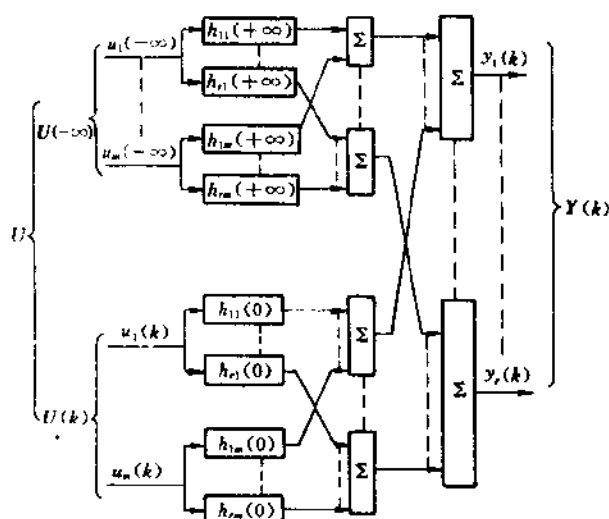
图 1-5 有 m 个输入、 r 个输出的多变量系统中，输入输出的关系
