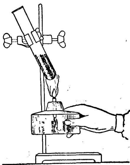
圖 4 硫化鐵的制取
