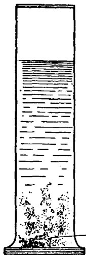
圖2 高錳酸鉀在水中的扩散
