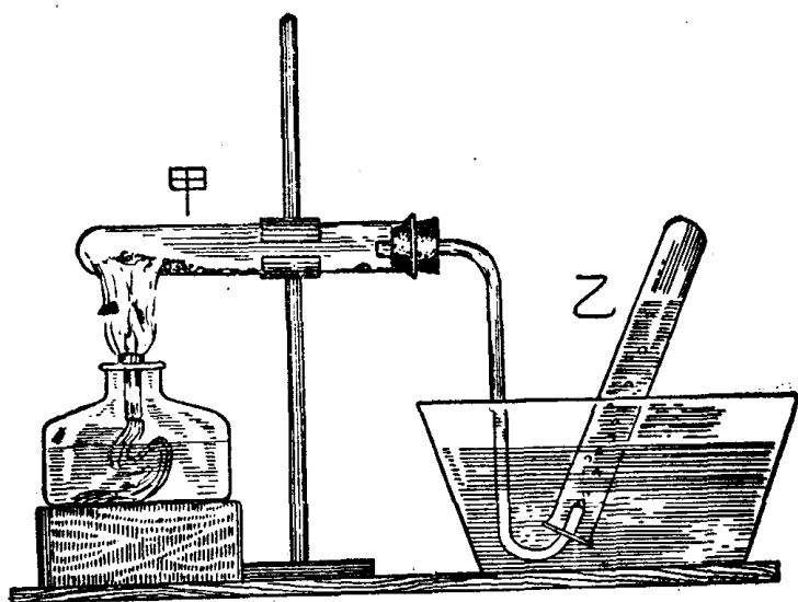
圖 3 氧化汞的分解
