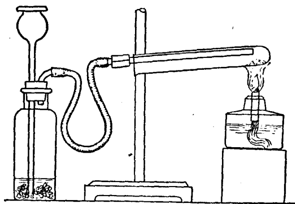
圖5 氧化銅的還原
