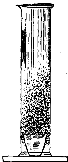
圖1 溴气在空气中的扩散
