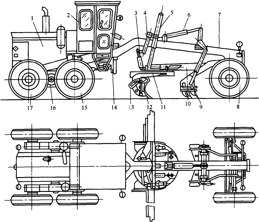
图 1-4 平地机结构
