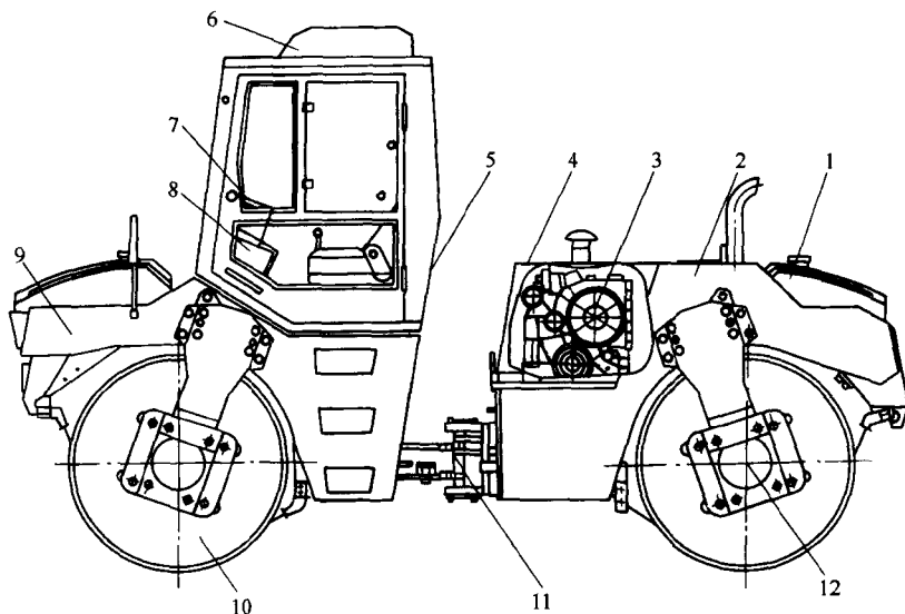
图 1-7 压路机结构
