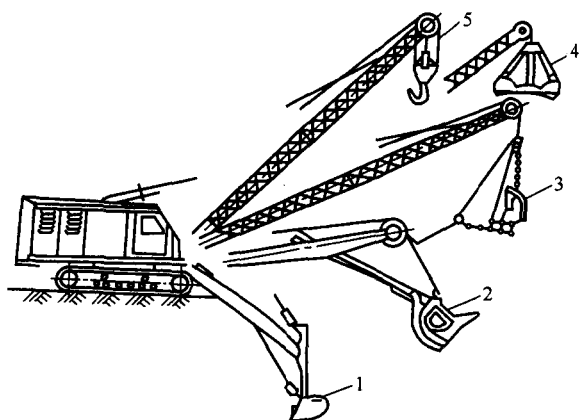
图 1-1 单斗挖掘机工作装置
