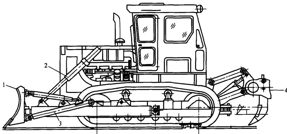
图 1-2 推土机结构
