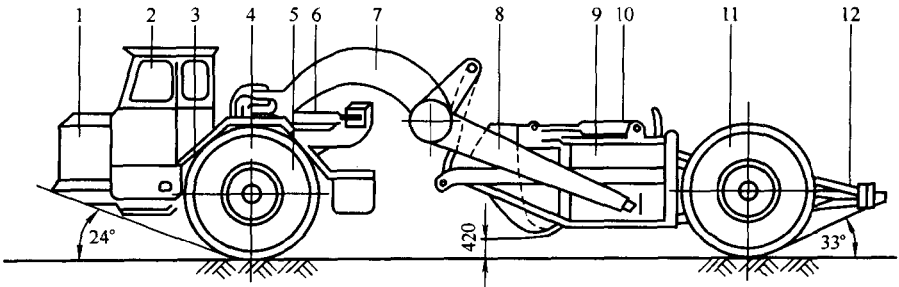
图 1-3 自行式铲运机
