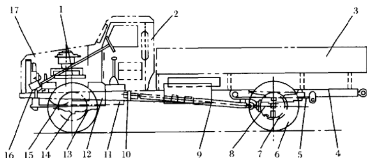
图 1-3 汽车的总体构造
