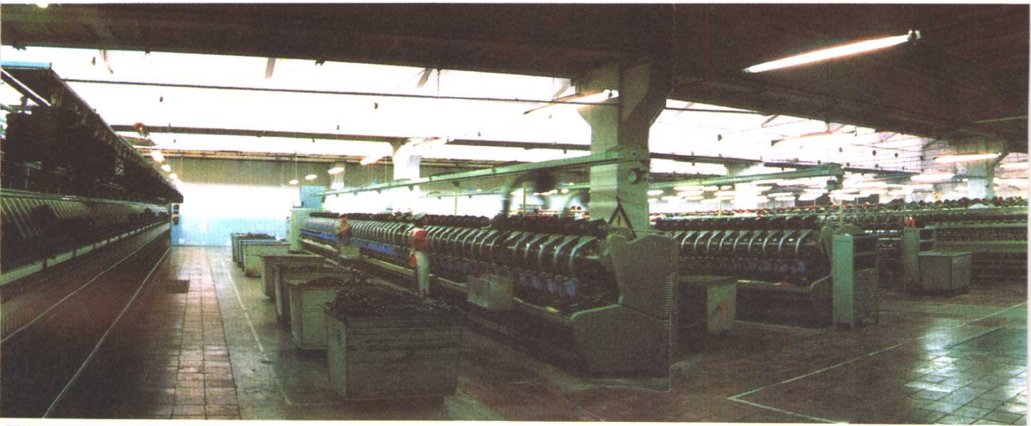
内蒙第二毛纺织厂 4800锭新车间
