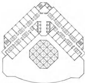
标准层平面
