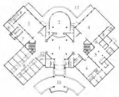
一层平面
