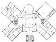
二層平面
