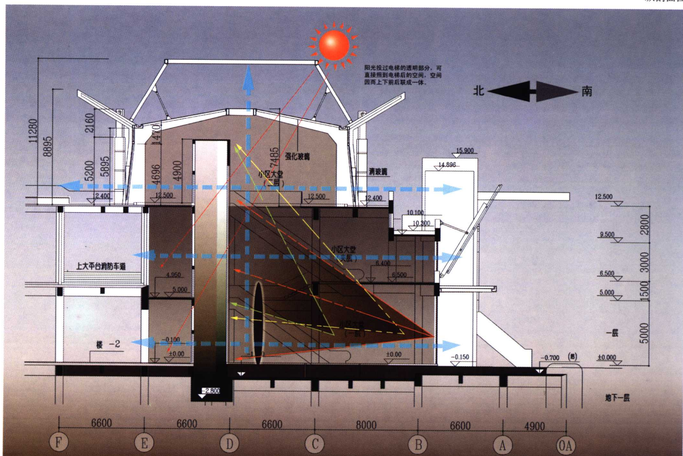
纵剖面图
