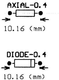
图1-5 两种相似的封装
