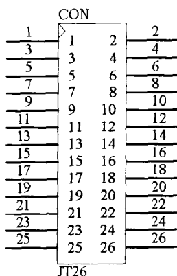
图1-2 26针双排塑料插座的原理图符号 2
