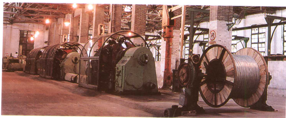
间一角。 ▶福州电线厂生产架空线的车
