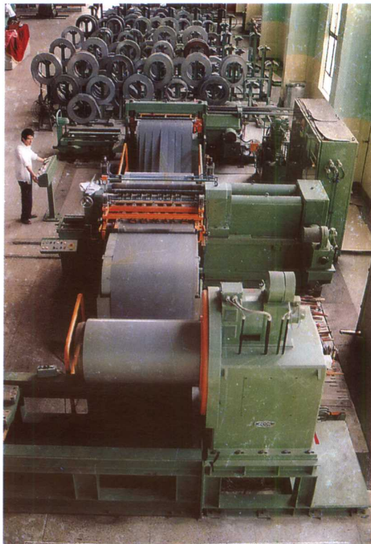
▲福州变压器厂引进德国 GEORG 公司硅钢片纵剪切线。
