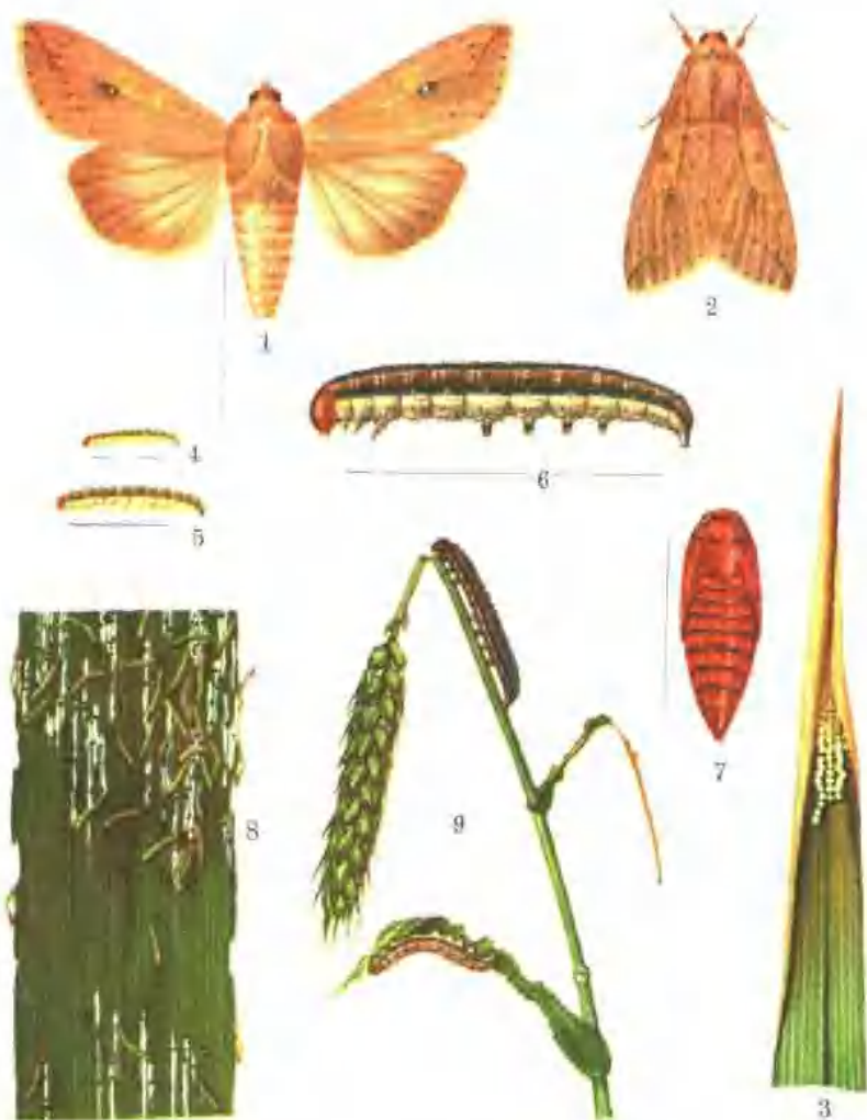
图版 3-7 粘 虫
