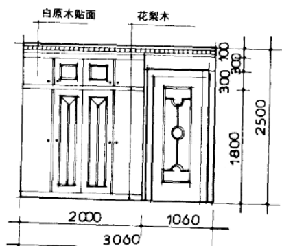
夫妇卧房 B 立面
