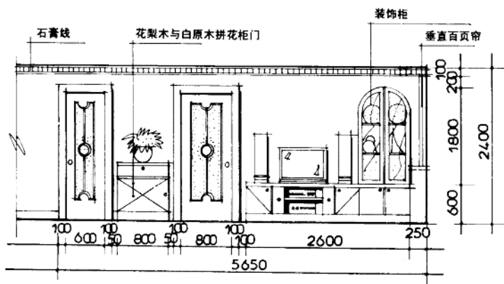
客厅C立面
