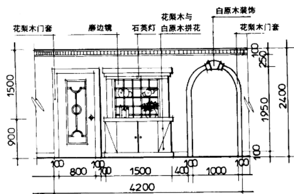
客厅B立面(酒柜)
