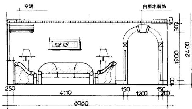
客厅A立面
