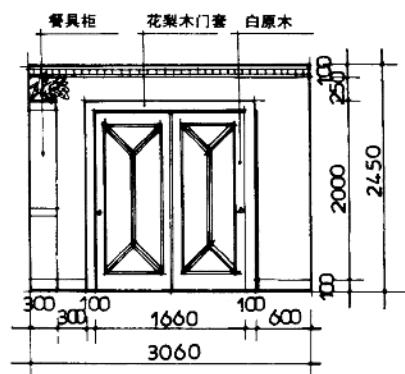
餐厅B立面
