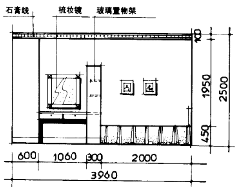
儿童房A立面
