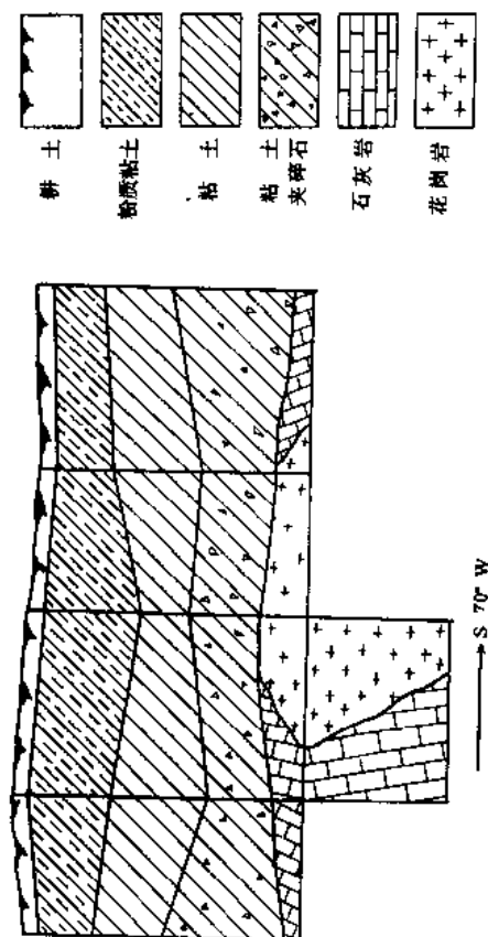
附录 E 探井展开图式
