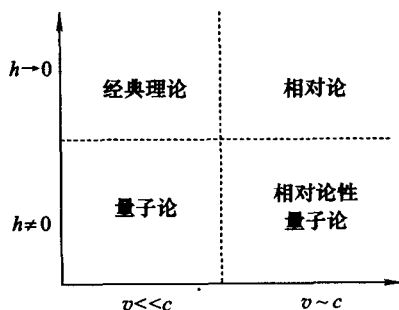
图 0-1-1 按物理常数 c 、 h 分类的物理学
