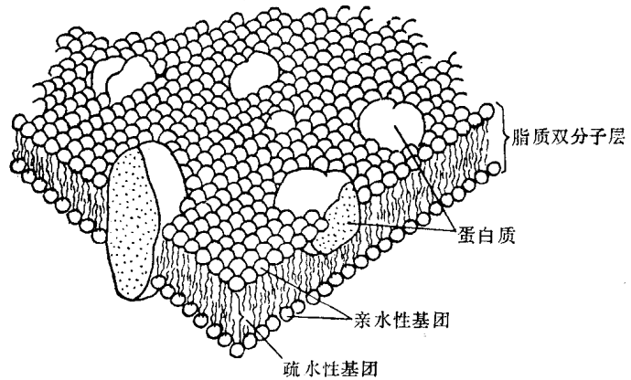
图 2-2 单位膜的液态镶嵌式模型
