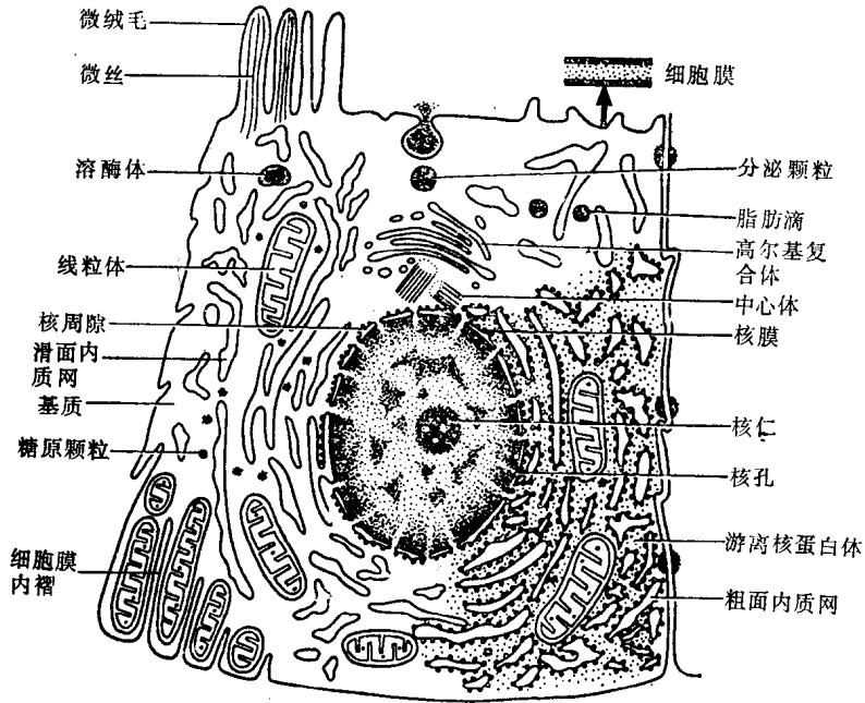
图 2-1 细胞超微结构模式图
