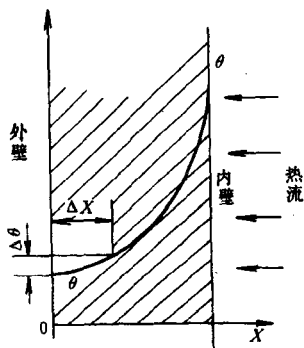
图 1-1 汽包壁内 温度变化图
