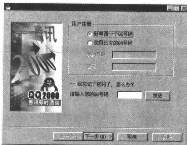
图 1.9 注册向导
