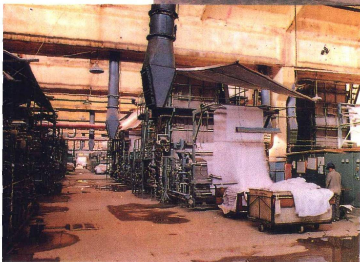
◀唐山印染厂漂洗车间流水线作业线。
