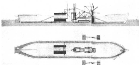
菲尔德所绘的汽船设计图
