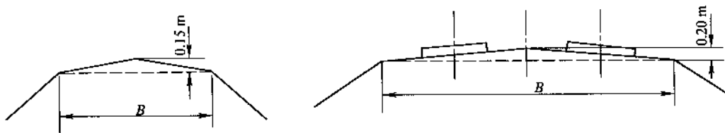
图2-3 单、双线路基路拱图
