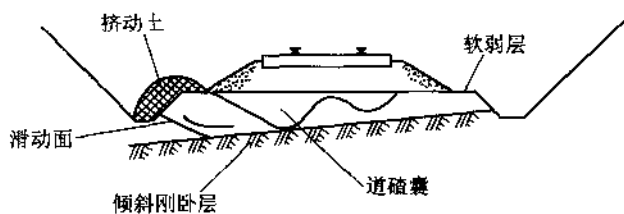
图 1-2 基床外挤
