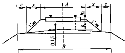
(a)单线非渗水土路基面宽度
