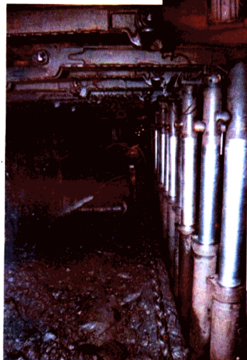
三矿井下单体液压支架工作面
