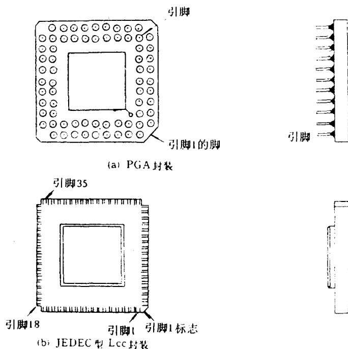
图 1-1 80286 微处理器
