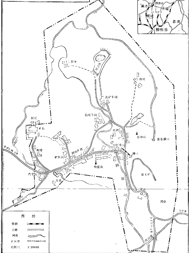
泗顶铅锌矿区平面图
