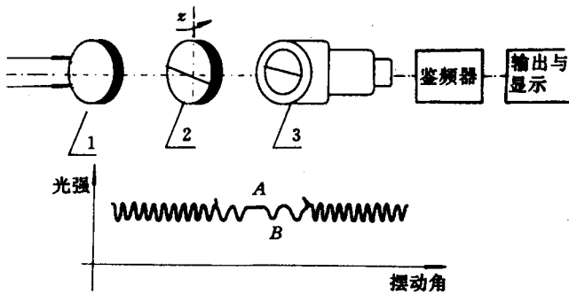
图 0-11 法布里-泊罗干涉仪型
