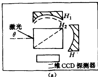
(a)图为原理图,(b)图为探测到的干涉图形 图 0-12 迈克尔逊相干识别型激光告警器
