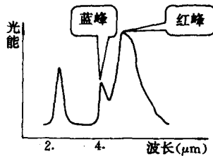
图 0-7 尾焰的波谱曲线图
