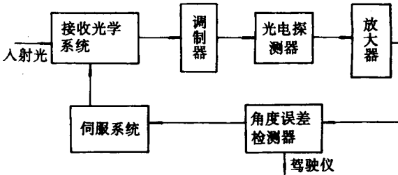
图 0-2 红外导引头原理方块图
