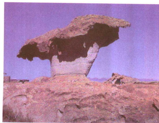
3. 磨菇石
