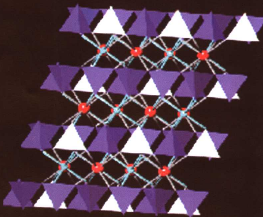
2. 链状角闪石
