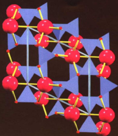
1. 架状长石
