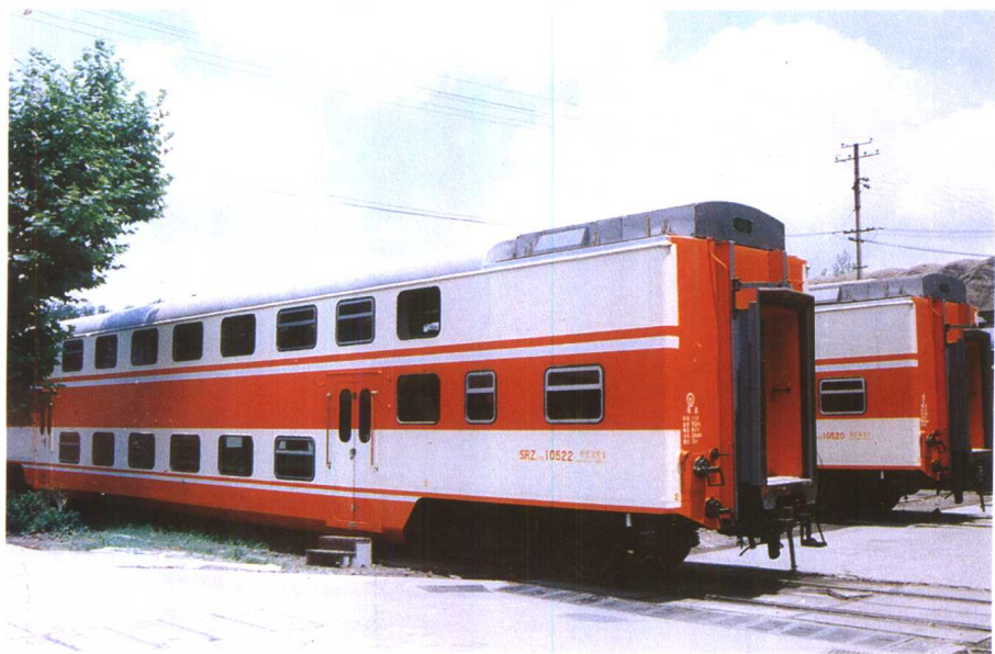
▲南京浦镇车辆厂研制生产的国内首列双层空调软座车
