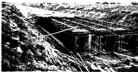
黄浦江上游引水工程三孔总管在现场扎筋浇注
