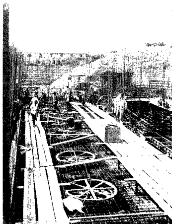
施工中的南区污水泵站
