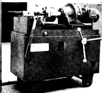
▲栋梁牌 XZL—40 型钢筋锥螺纹机床
