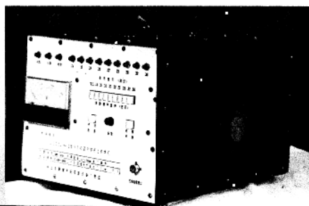
▼栋梁牌 LDZ—3—36 型电渣焊机(控制箱)
