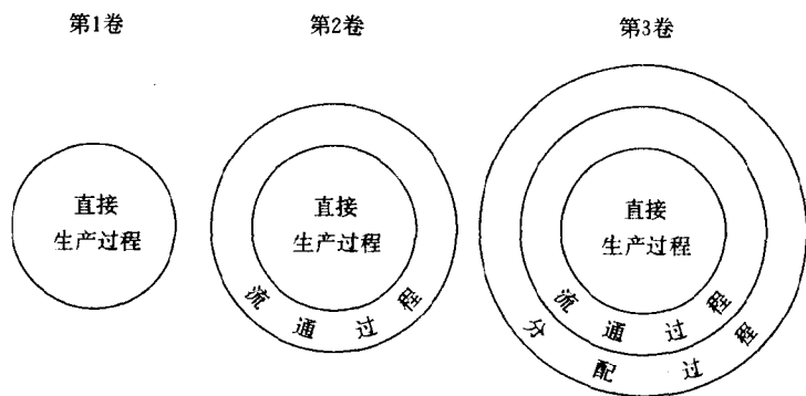
图0.1 圆圈表述法
