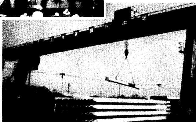
建筑构件公司 生产的钢筋混凝土 方桩和予应力钢筋 混凝土空心桩
