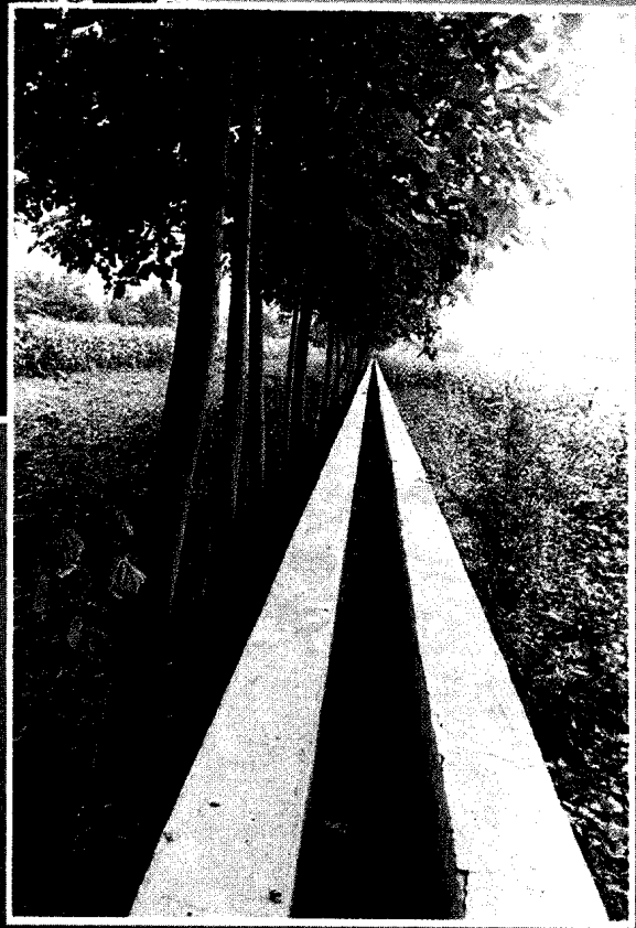
万金渠灌区硬化后的农田支渠
