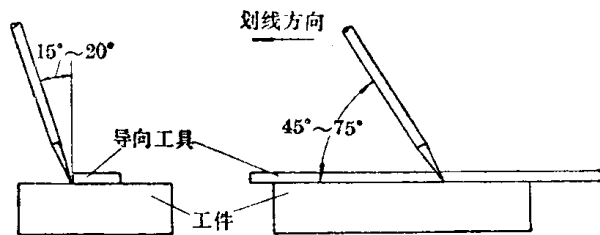
图 1-2 划针使用方法
