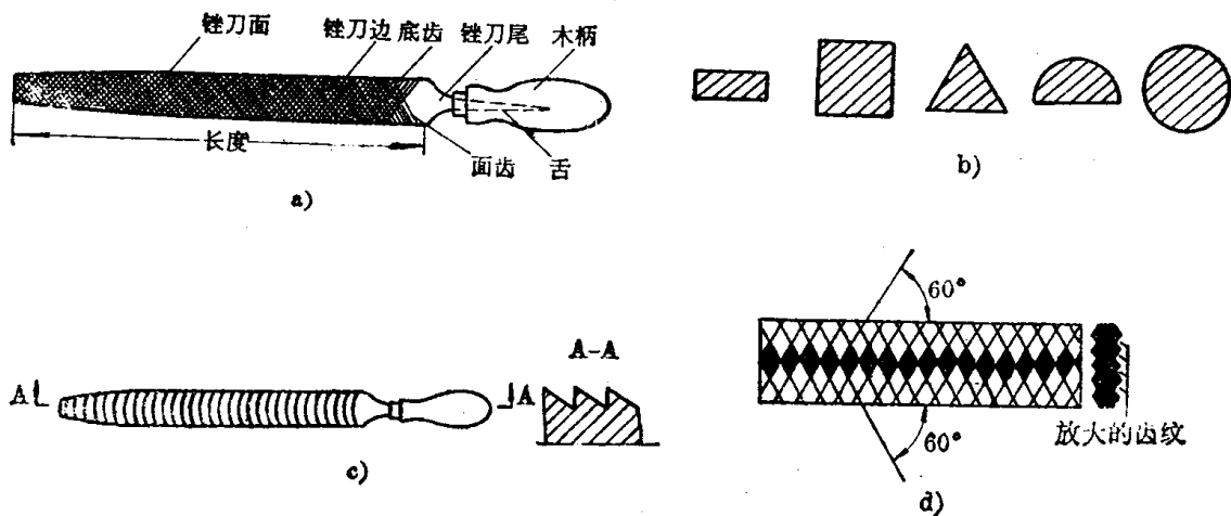
图 1-15 常用锉刀
