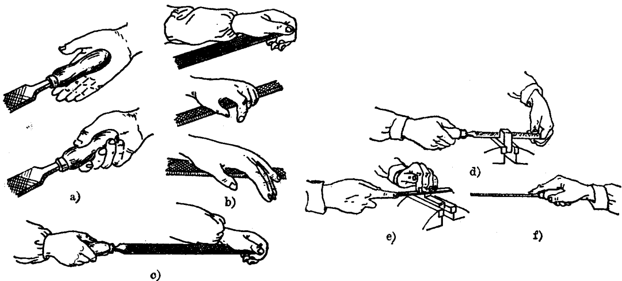
图 1-16 锉刀握法
