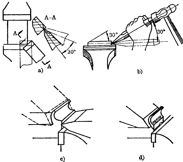
图 1-14 起凿和凿尽的方法
