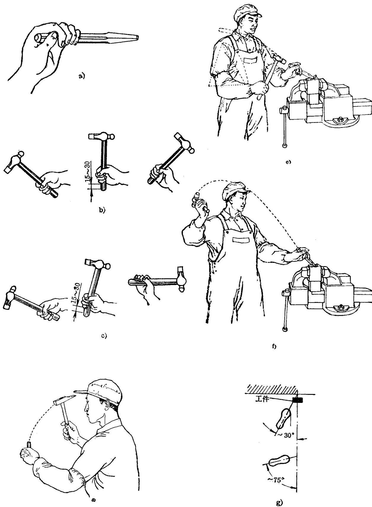
图 1-12 凿削的操作姿势
