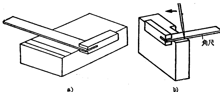
图 1-6 用靠边角尺划线
