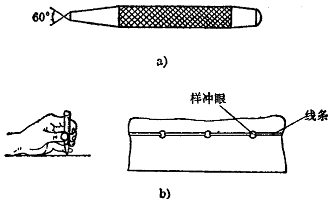
图 1-4 样冲
