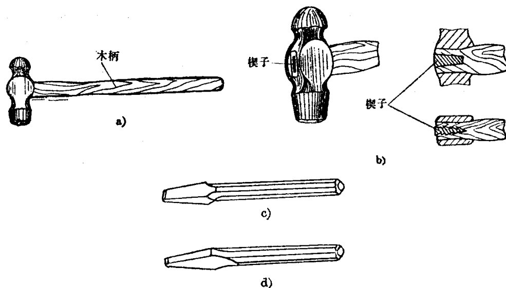
图 1-8 凿削工具
