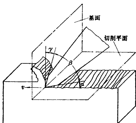
图 1-9 凿削时凿子的几何角度
