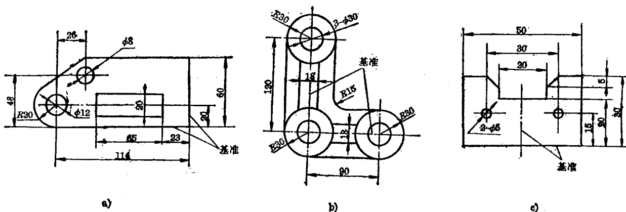
图 1-5 划线基准
