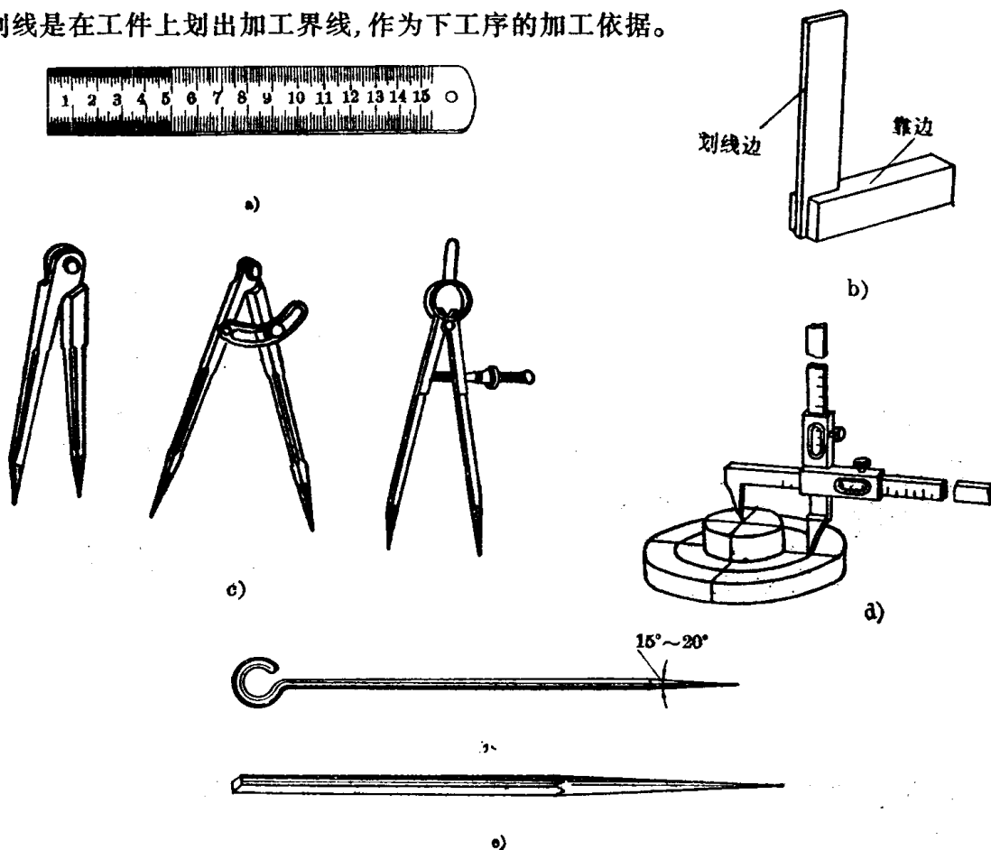
图 1-1 划线工具
