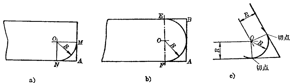
图 1-7 圆弧划法
