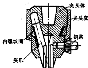
图 1-17 钻夹头
