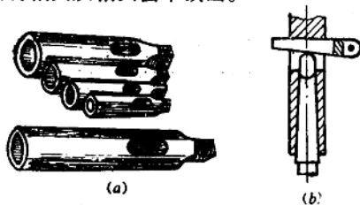
图 1-18 钻头套和钻头的拆卸
