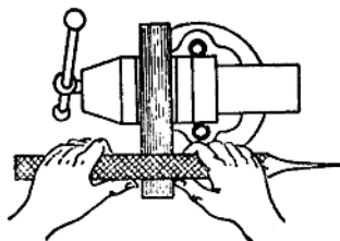
图 1-13 推锉
