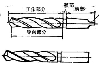
图 1-15 麻花钻 (a) 直柄；(b) 锥柄
