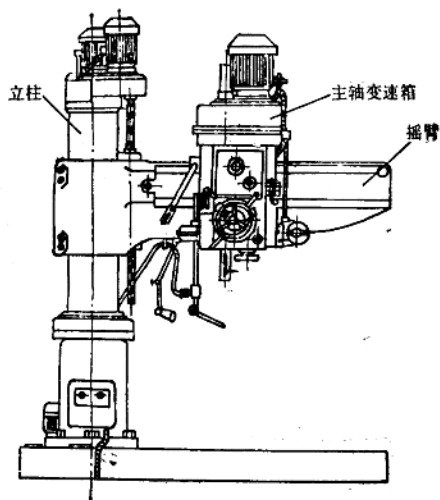
图 1-14 摇臂钻床
