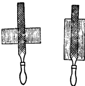
图 1-11 顺向锉
