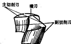
图 1-16 麻花钻的切削部分
