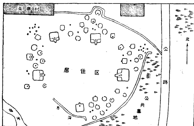
图一 姜寨氏族聚落遗迹平面图
