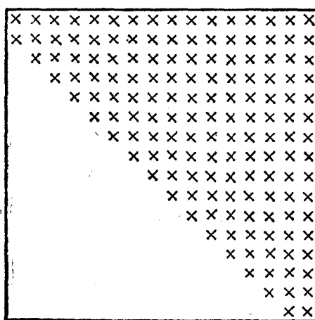
图 1.24 上海森堡矩阵
