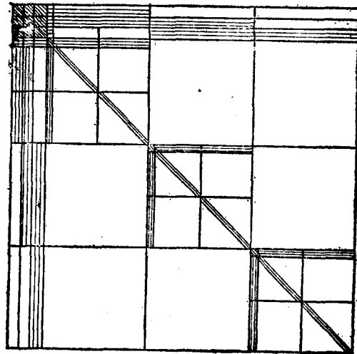
图 1.20 稀疏对称反向二重子结构矩阵
