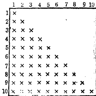
图 1.1 下三角阵
