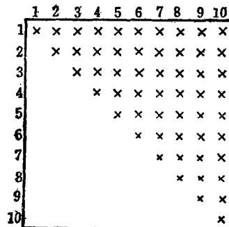
图 1.2 上三角阵
