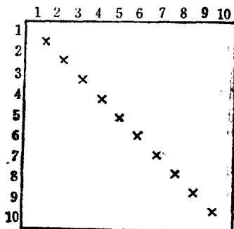
图 1.3 对角阵
