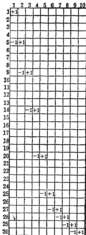
图 1.22 极稀疏长方带状矩阵
