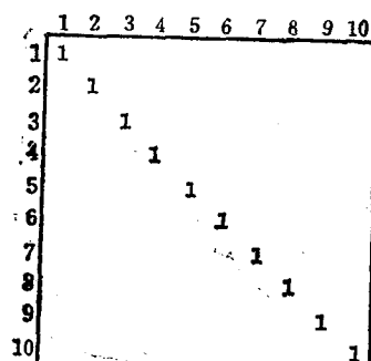
图 1.4 单位阵
