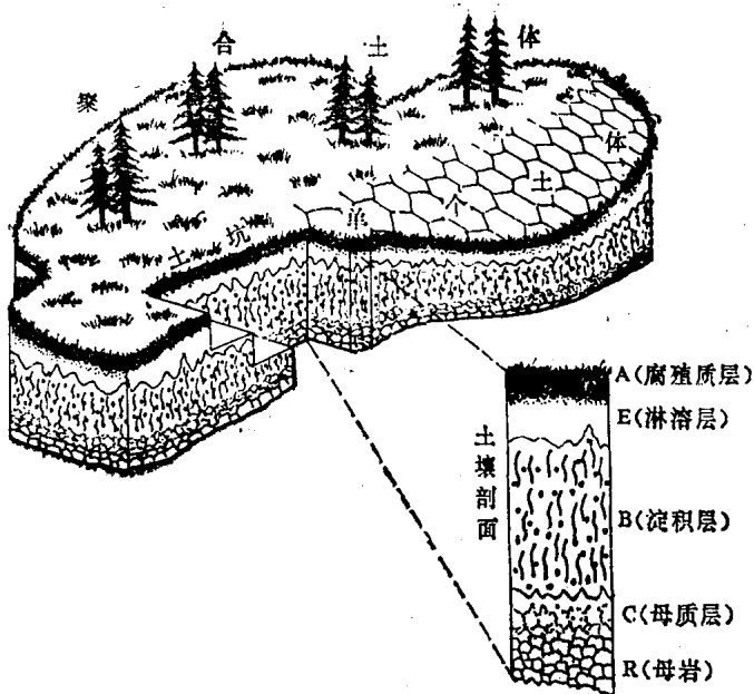
图 1-2 土壤剖面与单个土体、聚合土体三者之间的关系
