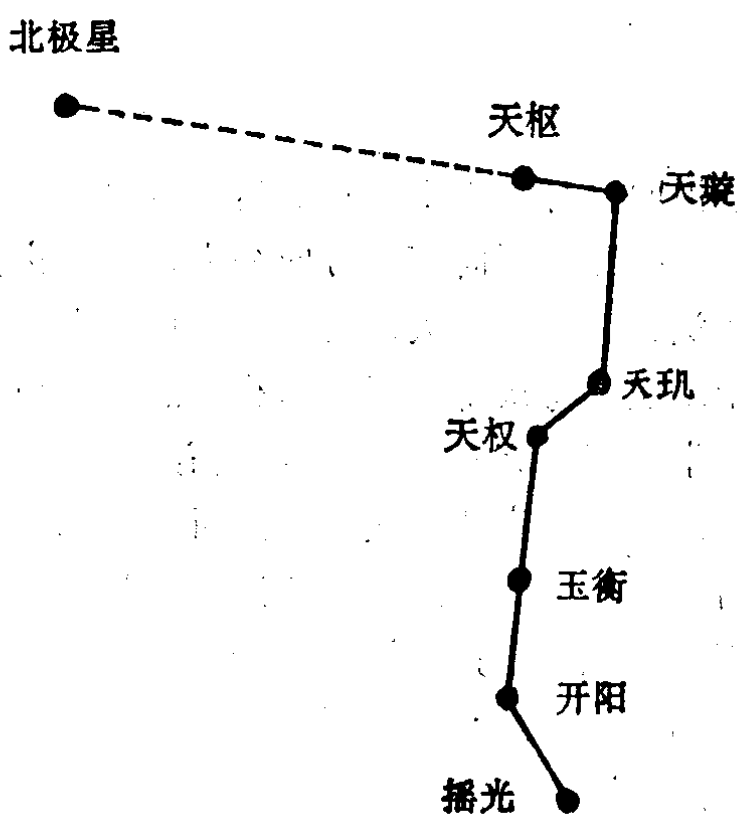
北极星图
