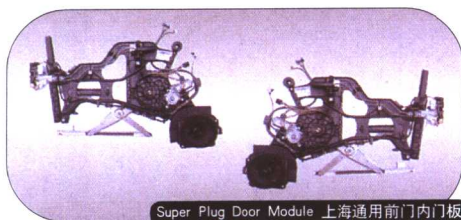
Super Plug Door Module 上海通用前门内门板
