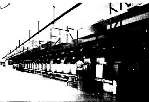
自行设计的现代化洗衣机装配流水线
