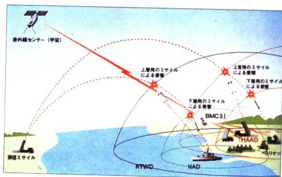
美国为日本设计的 TMD 示意图
