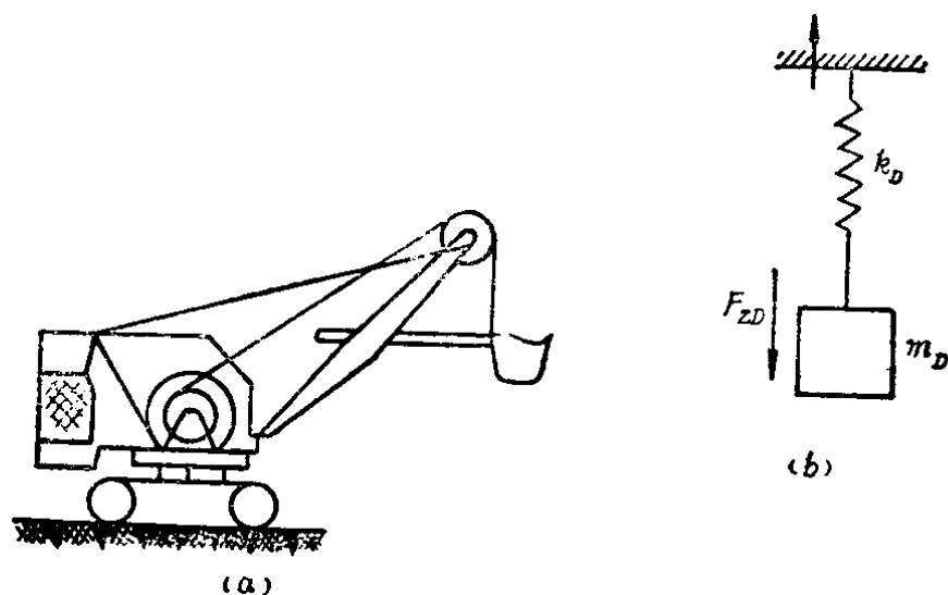
图 1—4 机械式单斗挖掘机简图
