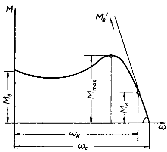
图 1—2 三相感应电动机的特性
