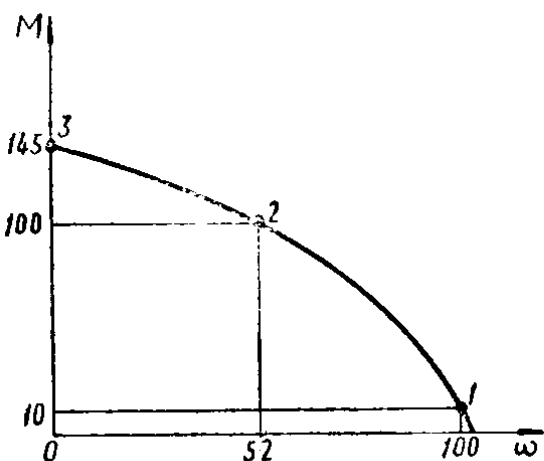
图 1—3 起重机用电机的特性
