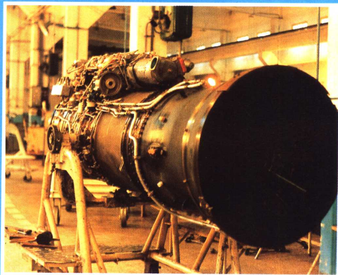
贵州航空发动机公司和成都航空发动机公司， 联合研制成功的涡喷——13航空发动机，于1987 年12月 1日通过国家级技术鉴定。（黎阳公司黄振国提供）
