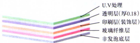
巴利斯 PVC 卷材的结构组成(总厚度 1.5)
