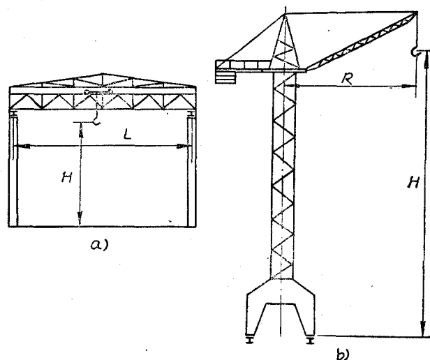
图 1-1 起重机跨距、幅度、起升高度示意图 a) 桥式起重机； b) 塔式起重机
