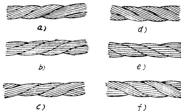
图 2-2 钢丝绳的捻制外形
